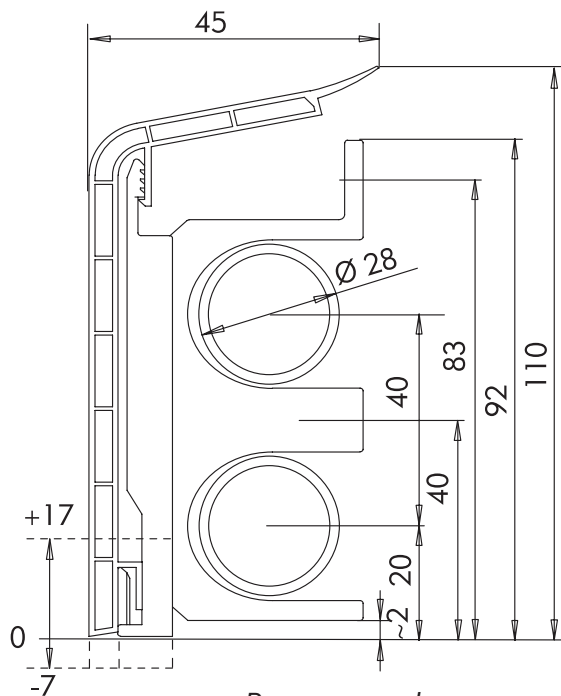
Размеры профиля и зажима для труб MIANO
