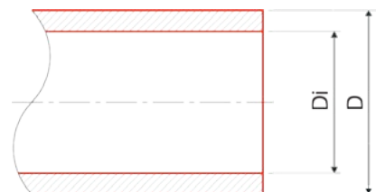
Размеры трубы FV PP-RCT UNI
